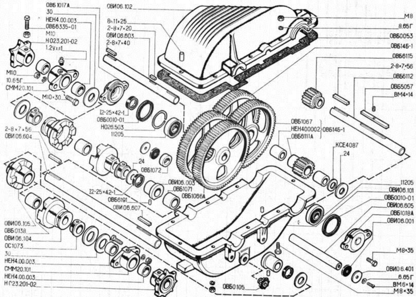
Рис. 29. Редуктор ОВИ 06.100.
